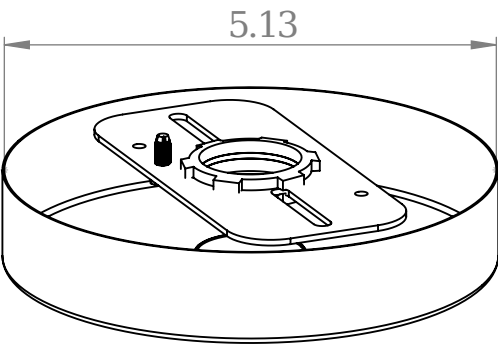
640-50 - 1/2" NPT CANOPY
