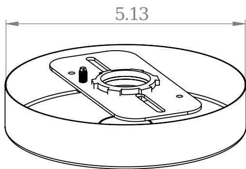
640-50 - 1/2" NPT CANOPY
