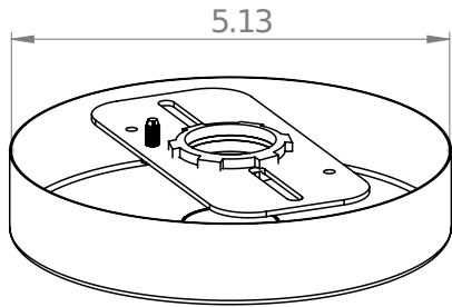
640-50 - 1/2" NPT CANOPY
