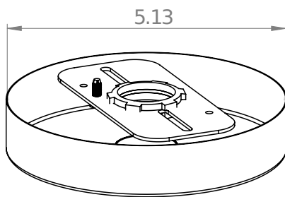
640-50 - 1/2" NPT CANOPY
