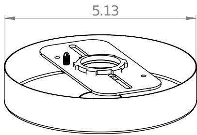
640-50 - 1/2" NPT CANOPY
