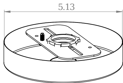
640-50 - 1/2" NPT CANOPY
