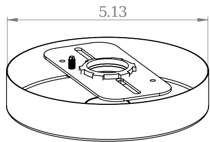
640-50 - 1/2" NPT CANOPY
